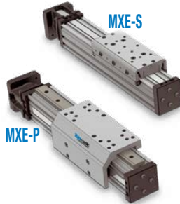
MX: Accionadores sin vastago con transmisión por tornillo de bolas, potencia neumática y correas
